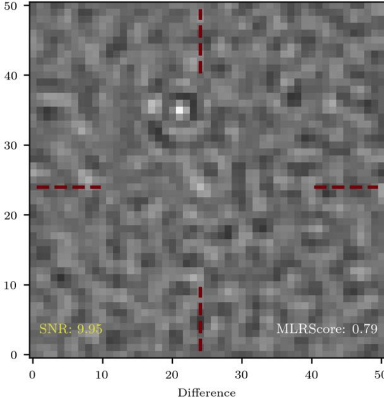
Sloan-i 25.15 [0.109] mag
